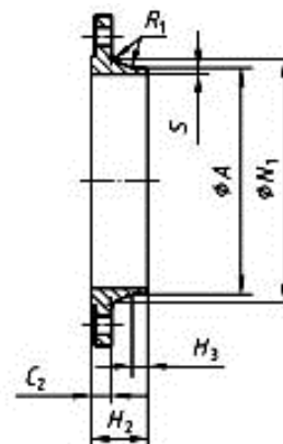
Type 11
