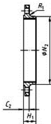
Type 13
