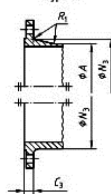
Type 11
