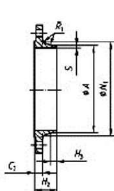
Type 11
